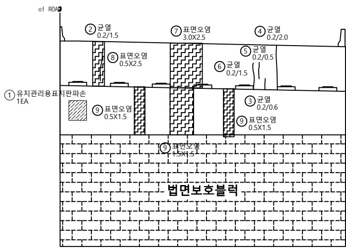
정면도
